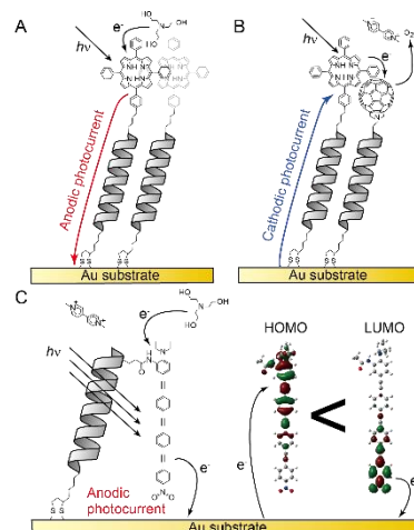
ペプチド SAM の光電変換特性
