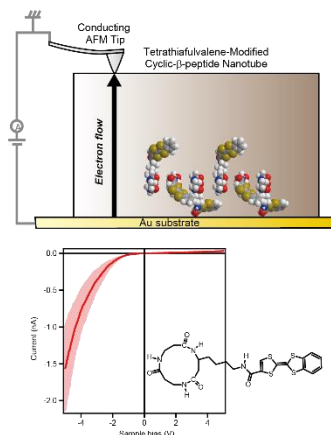
ペプチドナノチューブの電気的特性及び誘電体特性
